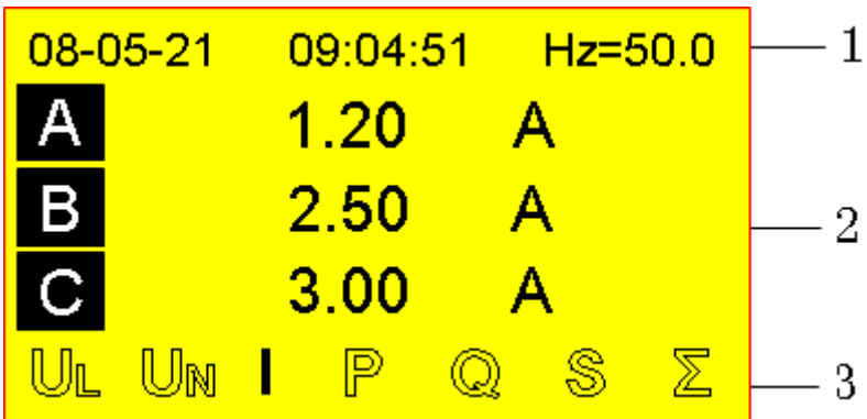
图 4.2.3-1 三相电流
