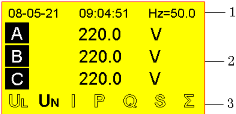
图 4.2.2-1 三相相电压
