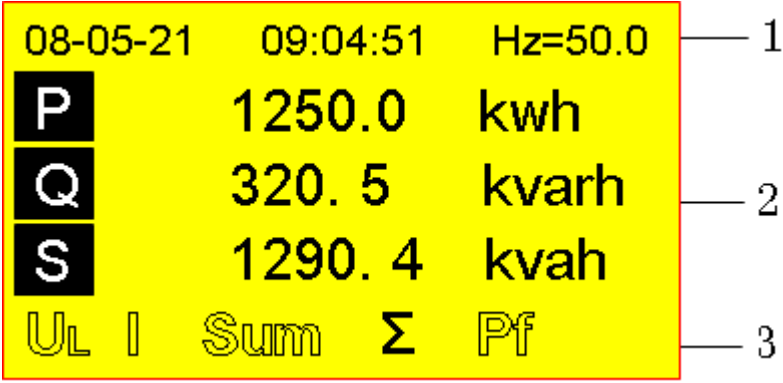
图 4.3.4-1 累计电能
