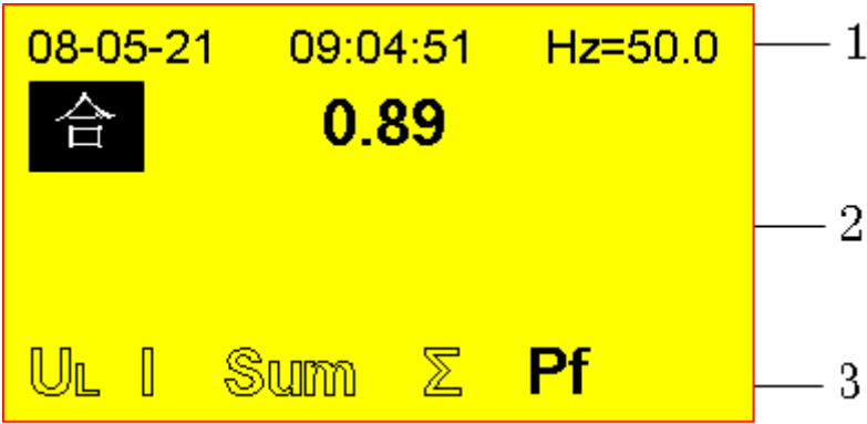
图 4.3.5-1 功率因数
