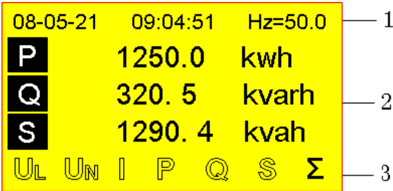
图 4.2.7-1 累计电能
