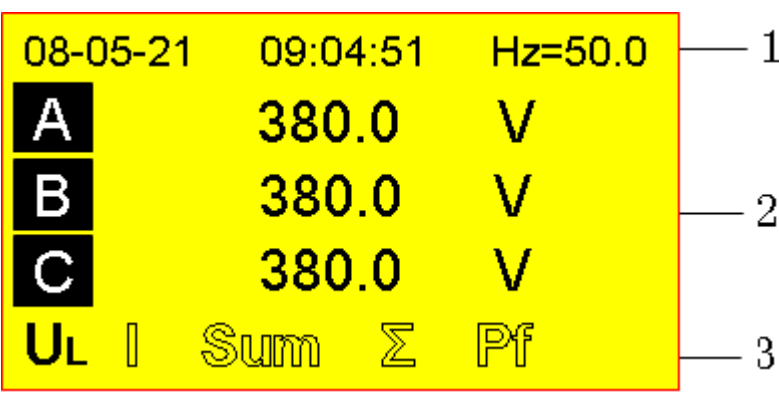
图 4.3.1-1 线电压
